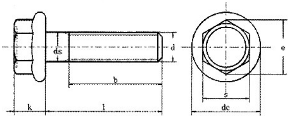
产品尺寸图
