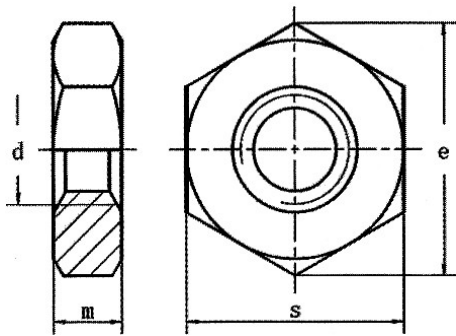
产品尺寸图
