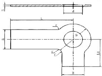
产品尺寸图
