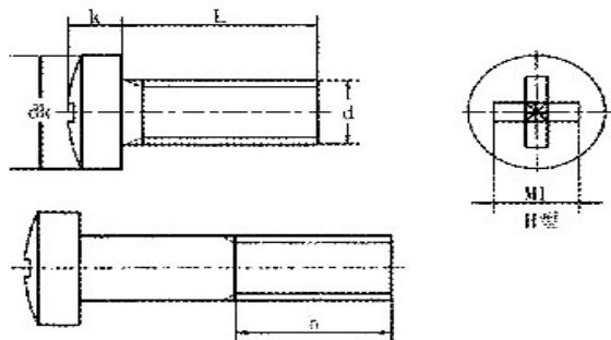
产品尺寸图
