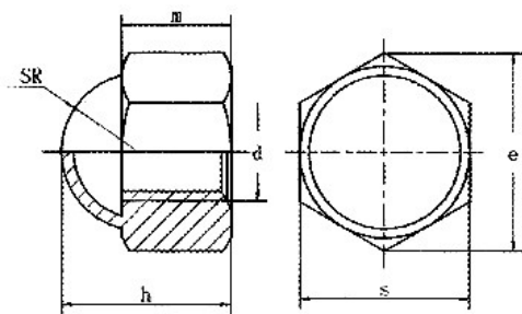
产品尺寸图
