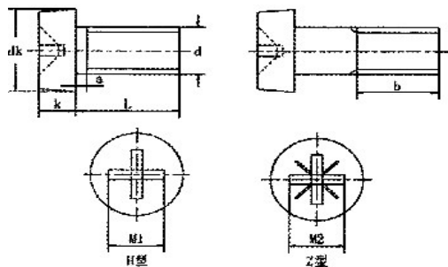
产品尺寸图
