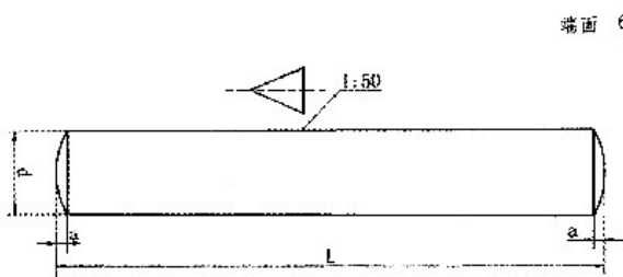
产品尺寸图
