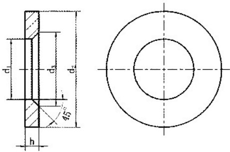
产品尺寸图
