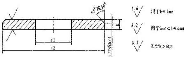
产品尺寸图
