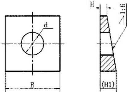
产品尺寸图
