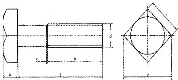
产品尺寸图
