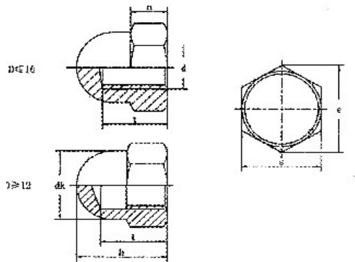
产品尺寸图
