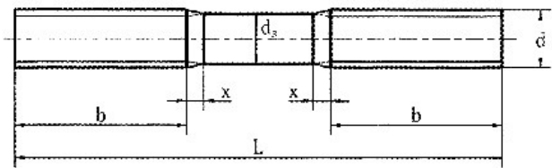
产品尺寸图
