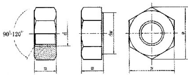
产品尺寸图
