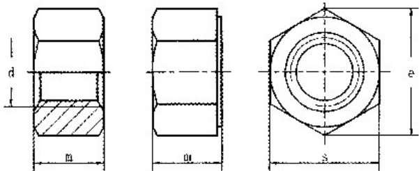
产品尺寸图
