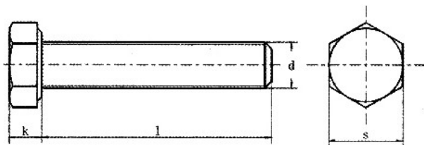
产品尺寸图
