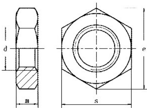
产品尺寸图
