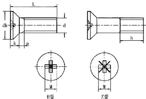
产品尺寸图
