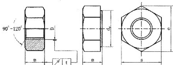
产品尺寸图
