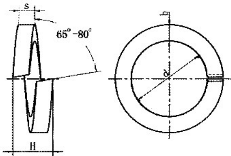
产品尺寸图
