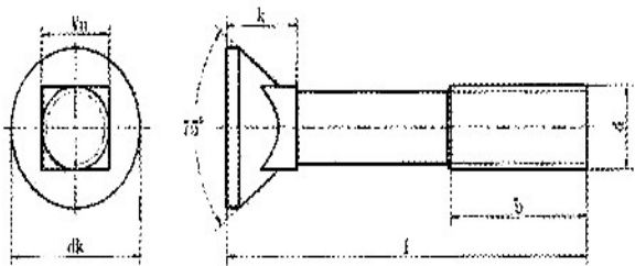
产品尺寸图
