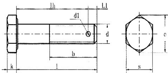
产品尺寸图
