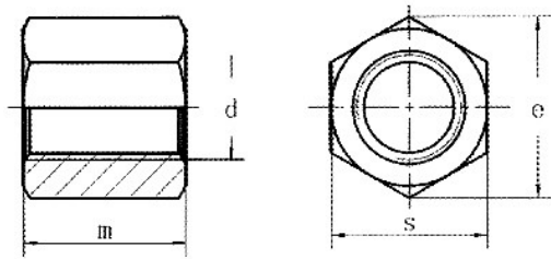
产品尺寸图
