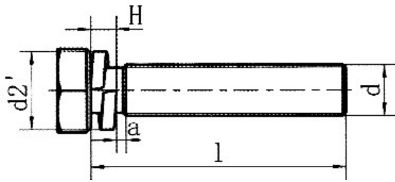
产品尺寸图
