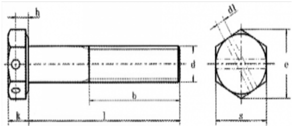
产品尺寸图
