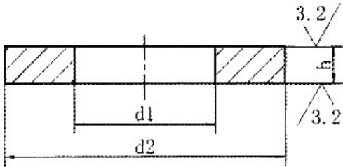
产品尺寸图
