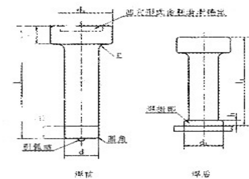
产品尺寸图
