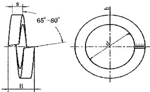
产品尺寸图
