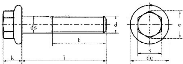
产品尺寸图
