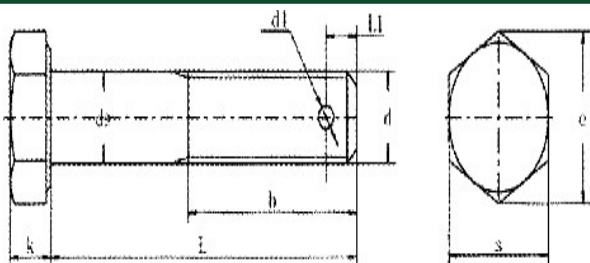
产品尺寸图
