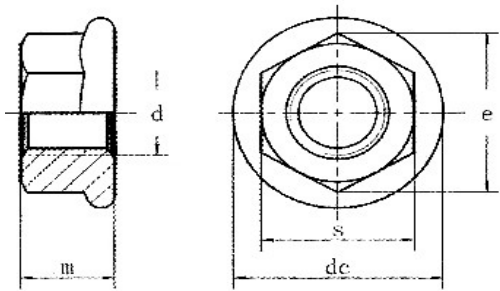
产品尺寸图
