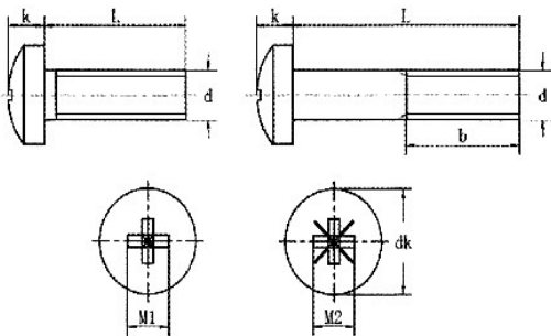
产品尺寸图
