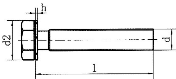
产品尺寸图
