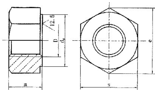
产品尺寸图
