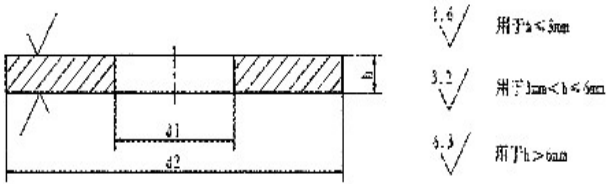
产品尺寸图
