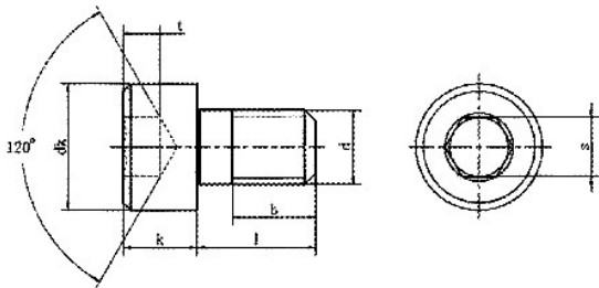
产品尺寸图
