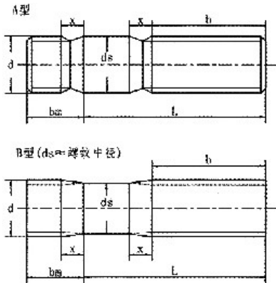
产品尺寸图
