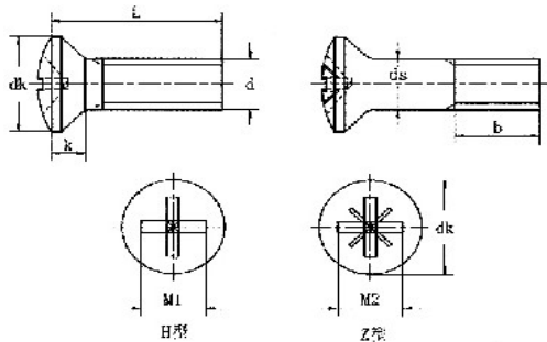
产品尺寸图
