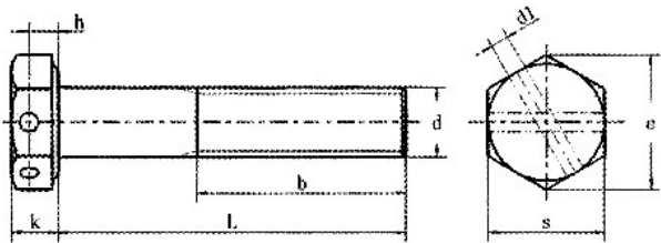
产品尺寸图
