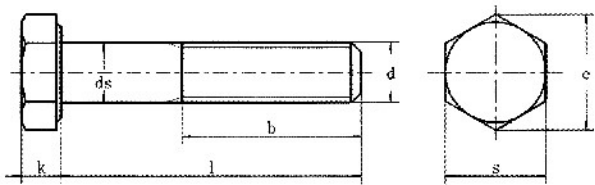
产品尺寸图
