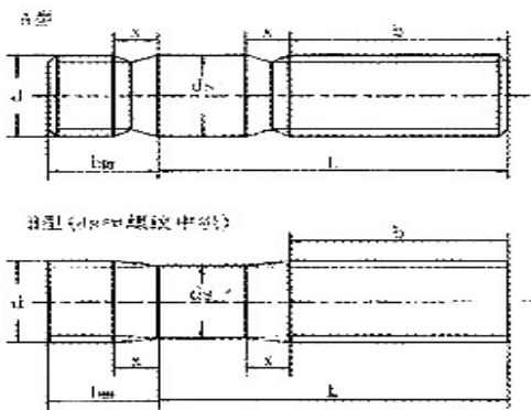
产品尺寸图
