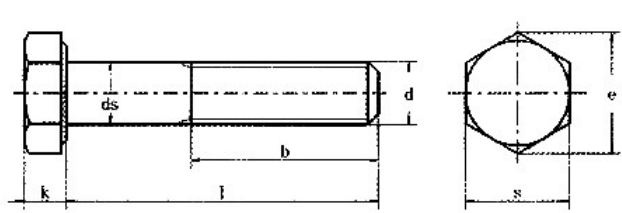
产品尺寸图
