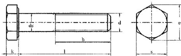
产品尺寸图
