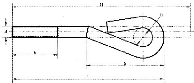
产品尺寸图
