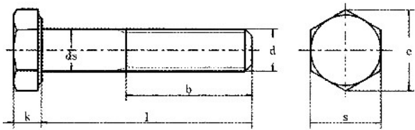
产品尺寸图
