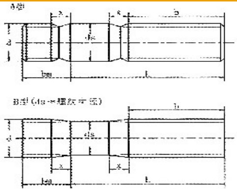
产品尺寸图
