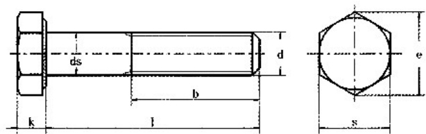
产品尺寸图
