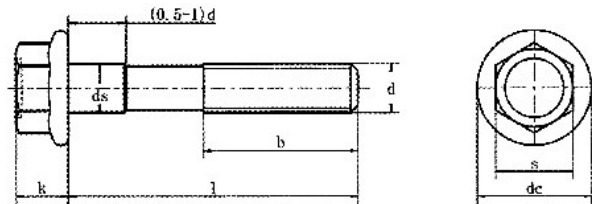
产品尺寸图
