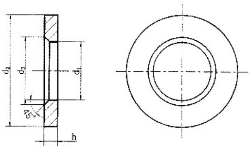
产品尺寸图
