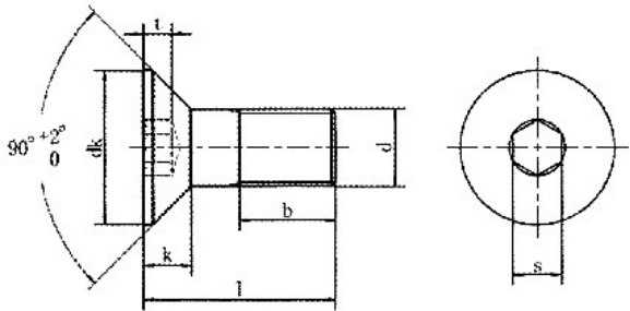
产品尺寸图
