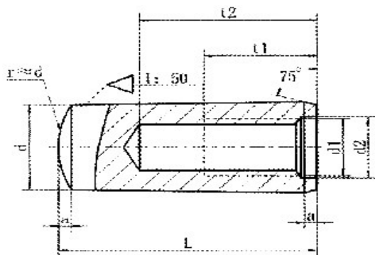
产品尺寸图
