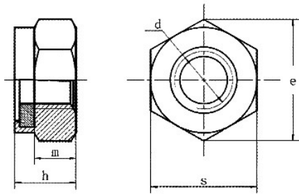
产品尺寸图
