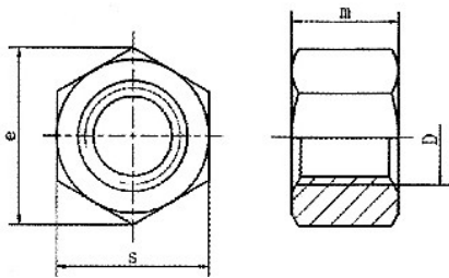
产品尺寸图
