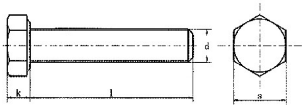
产品尺寸图
