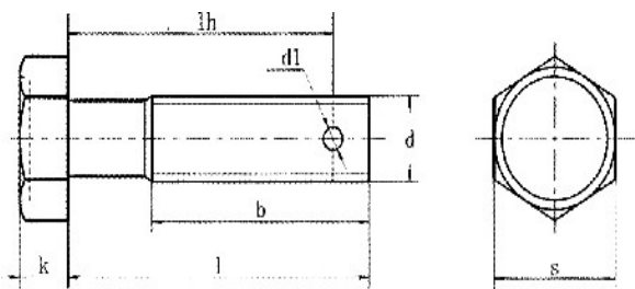
产品尺寸图
