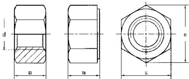
产品尺寸图
