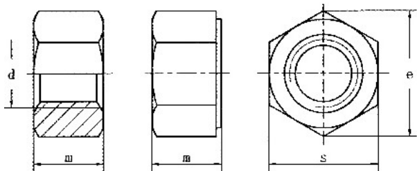
产品尺寸图
