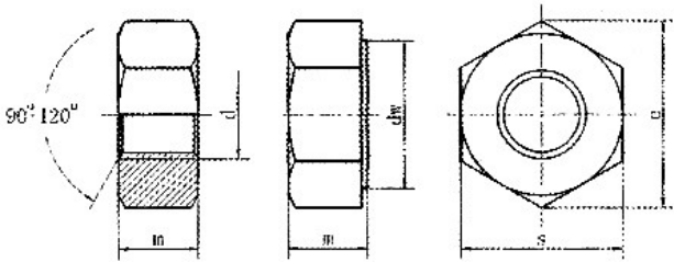
产品尺寸图
