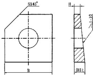
产品尺寸图
