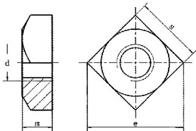
产品尺寸图
