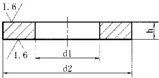
产品尺寸图
