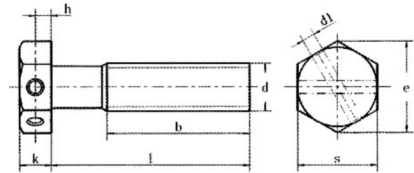
产品尺寸图
