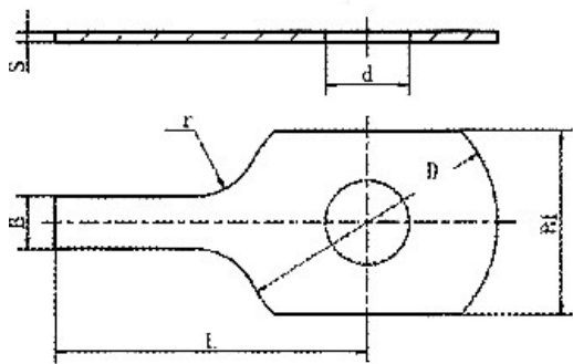
产品尺寸图
