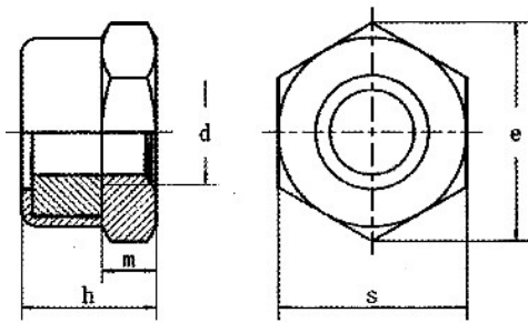
产品尺寸图
