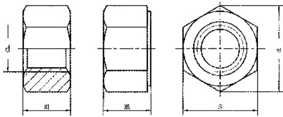
产品尺寸图
