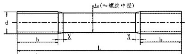
产品尺寸图
