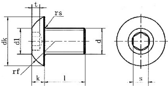
产品尺寸图
