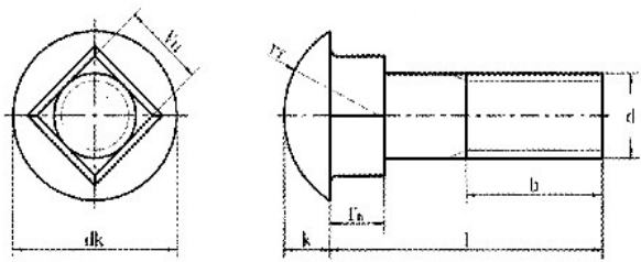
产品尺寸图
