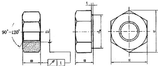
产品尺寸图
