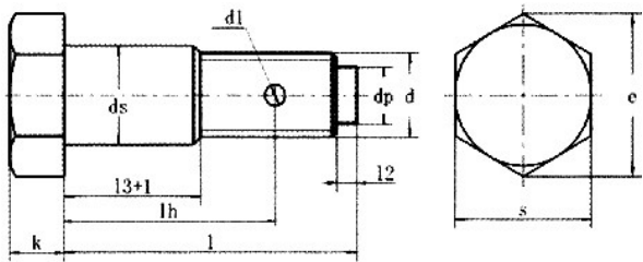
产品尺寸图
